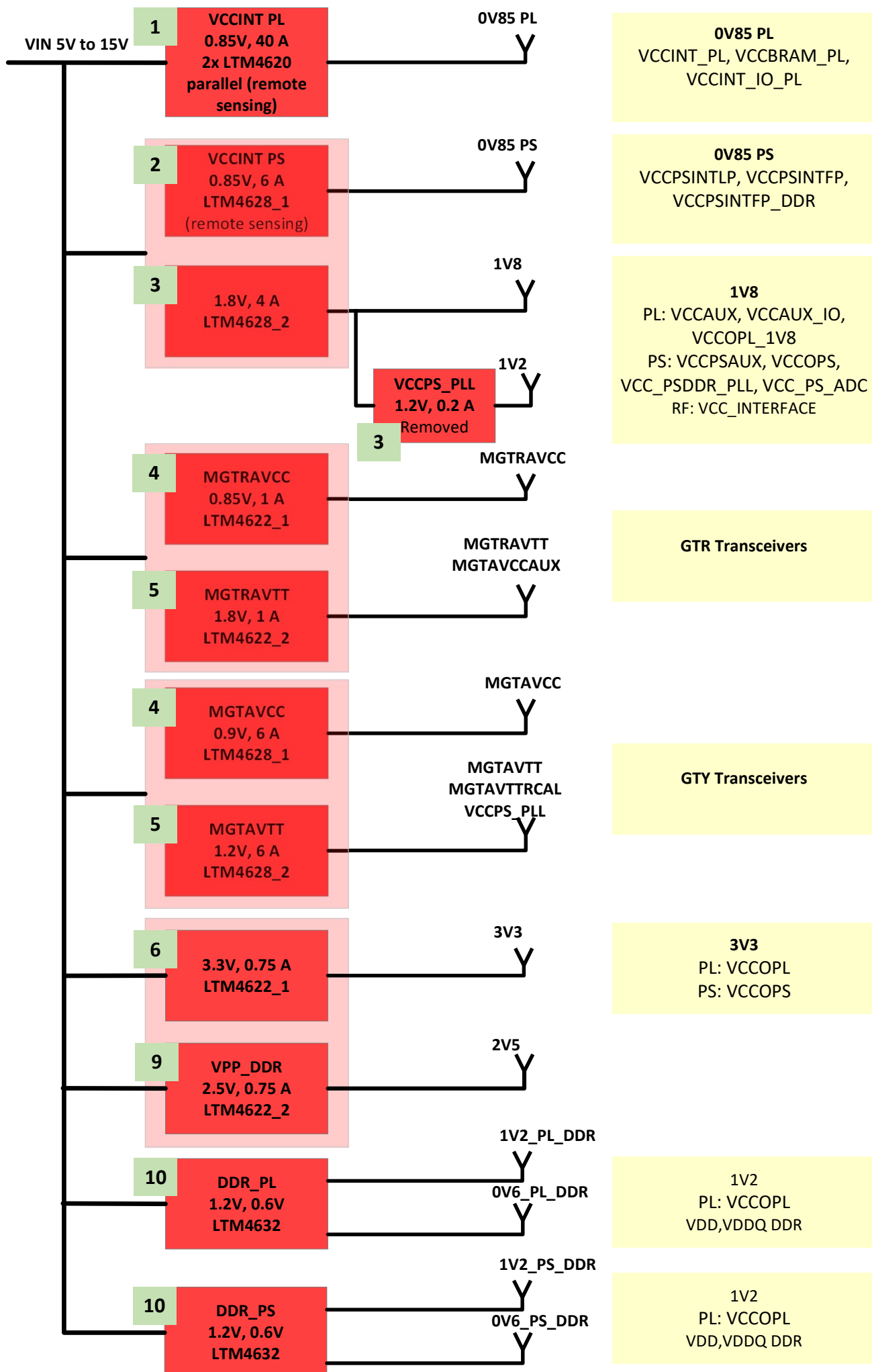
Talise SOM – ZYNQ Ultrascale Power Supplies
